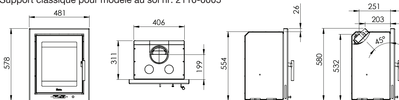
Support classique pour modèle au sol nr. 2110-0005
