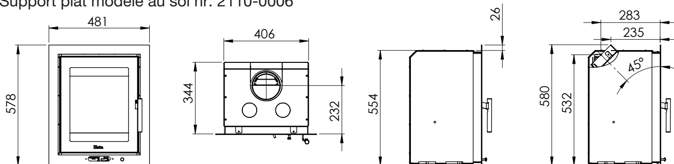
Support plat modèle au sol nr. 2110-0006
