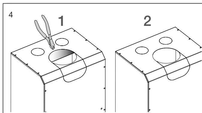
Sortie de fumée vers le haut.
