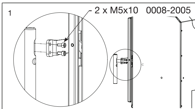
Montage de la poignée 0016-0031
