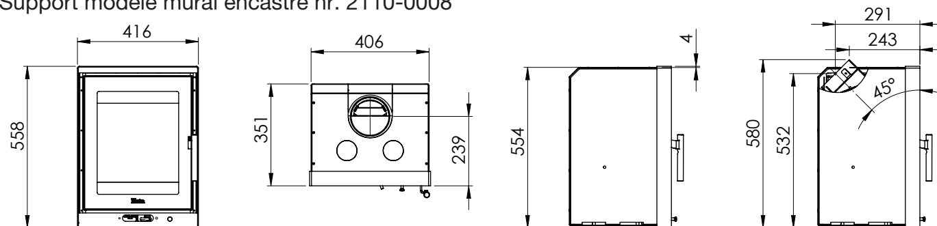
Support modèle mural encastré nr. 2110-0008
