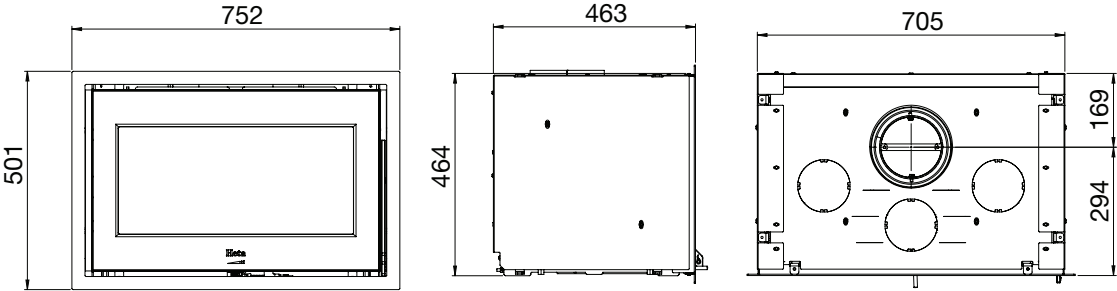
Schéma Prestige BR
