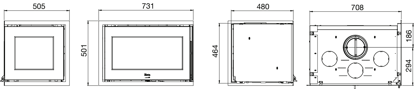
Schéma Prestige C
